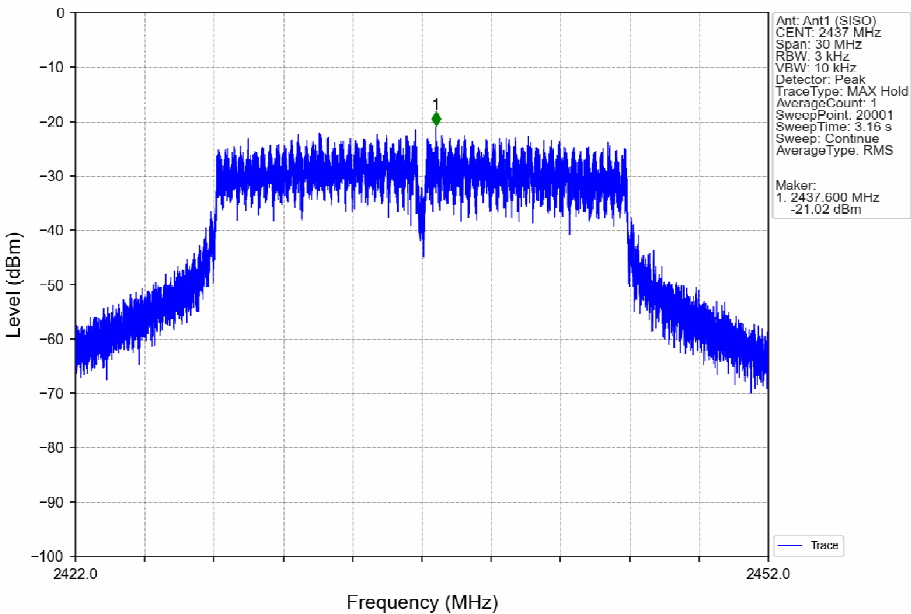
802.11n(HT20)_MCH_2437MHz_Ant1 (SISO)_NTNV
