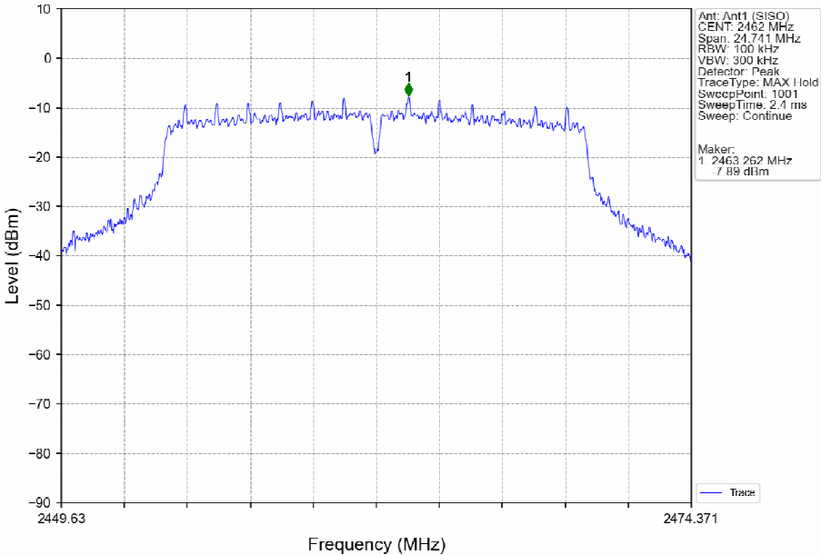
802.11g_HCH_2462MHz_Ant1 (SISO)_NTNV
