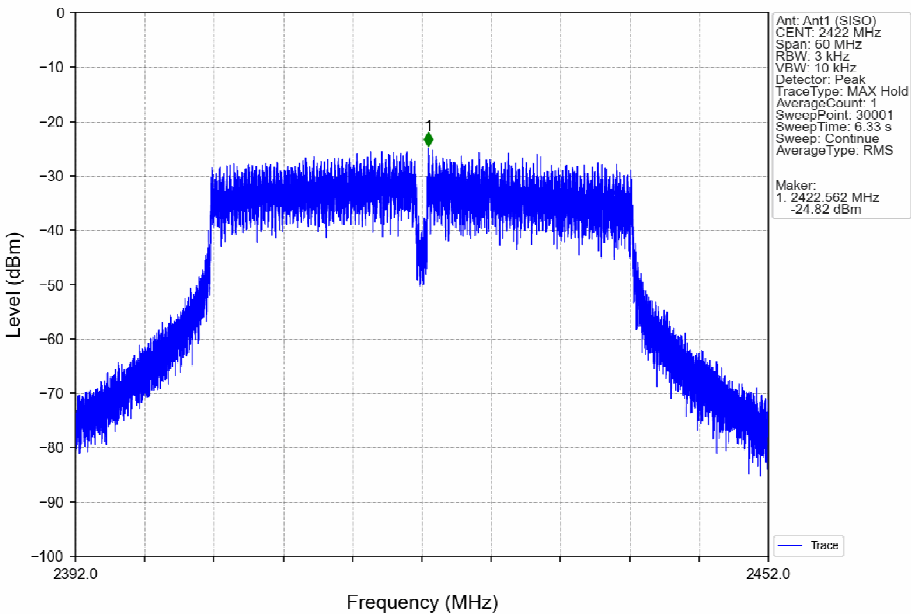
802.11n(HT40)_LCH_2422MHz_Ant1 (SISO)_NTNV
