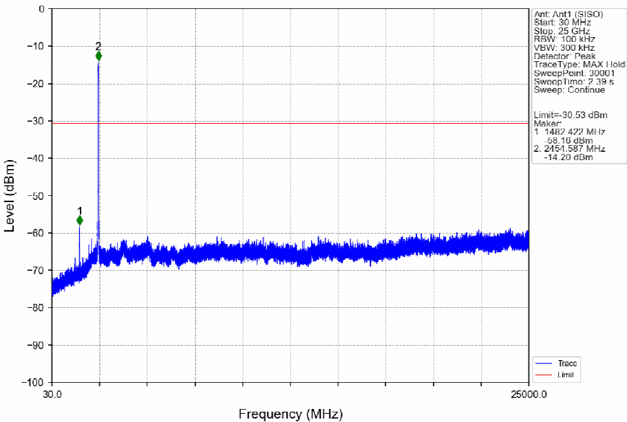
802.11n(HT40)_HCH_2452MHz_Ant1 (SISO)_NTNV
