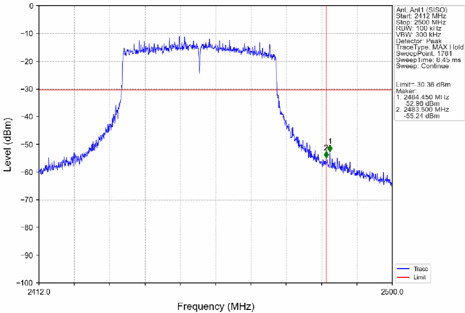
802.11ax(HEW40)_HCH_2452MHz_SU_/_Ant1 (SISO)_NTNV
