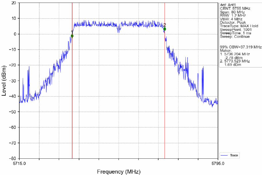
802.11n(HT40)_LCH_5755MHz_Ant1_NTNV
