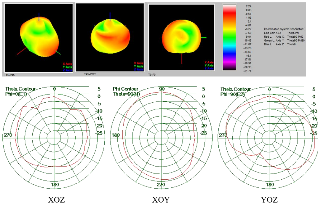
辐射方向图频率 315MHz
