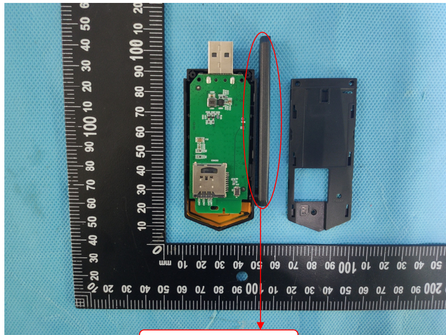
WCDMA/LTE ANT.
