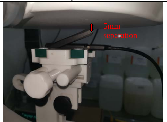
Bottom Side 45°
