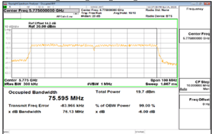
IC_802.11ac_80MHz_Chain1_5775MHz
