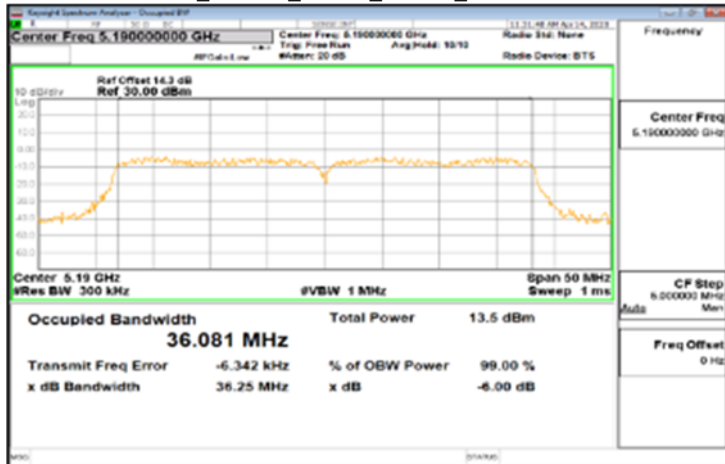
IC_802.11n_40MHz_Chain1_5190MHz
