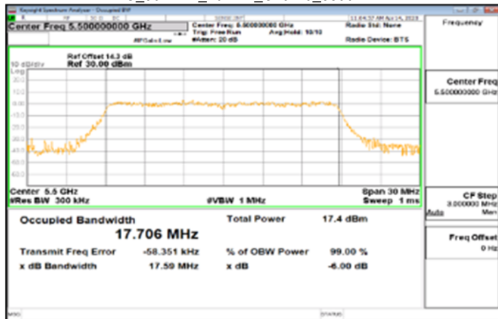
IC_802.11n_20MHz_Chain0_5500MHz
