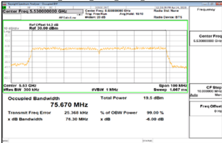
IC_802.11ac_80MHz_Chain1_5530MHz
