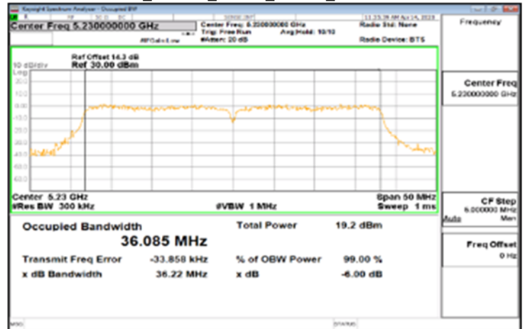
IC_802.11n_40MHz_Chain0_5230MHz
