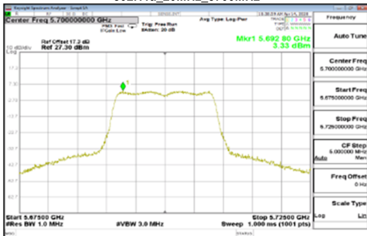
802.11a_20MHz_5700MHz
