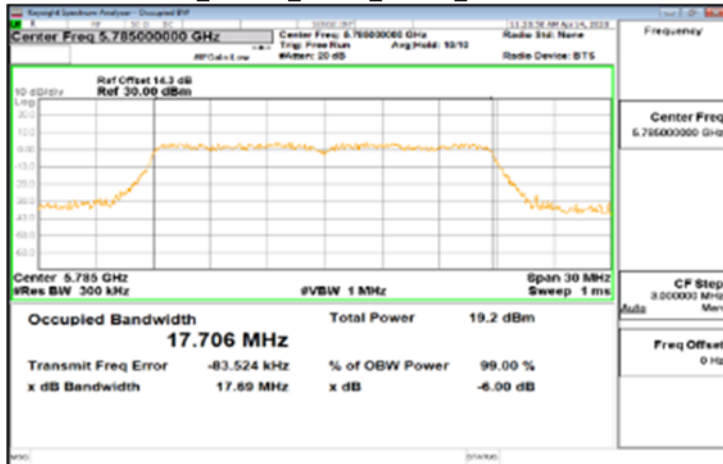
IC_802.11n_20MHz_Chain1_5785MHz
