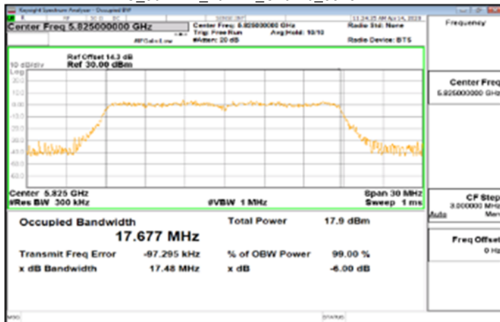
IC_802.11n_20MHz_Chain0_5825MHz
