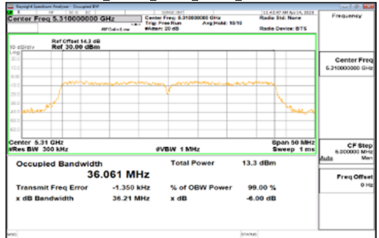
IC_802.11n_40MHz_Chain1_5310MHz
