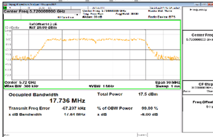
IC_802.11n_20MHz_Chain0_5720MHz
