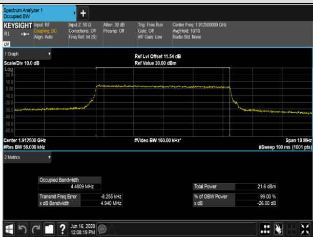
HCH_QPSK_25RB#0
