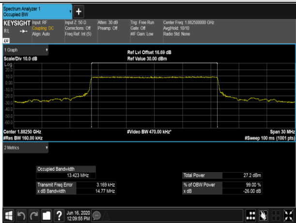
MCH_QPSK_75RB#0
