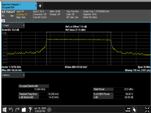
HCH_QPSK_75RB#0
