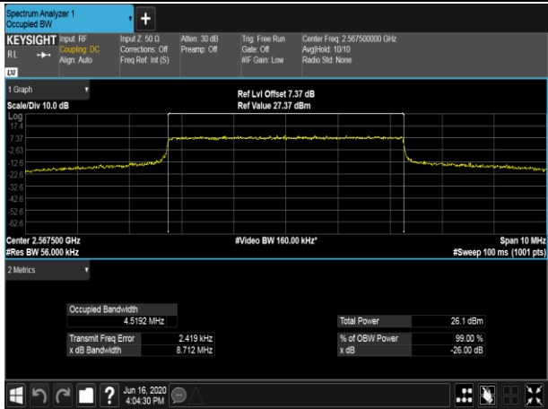
HCH_QPSK_25RB#0
