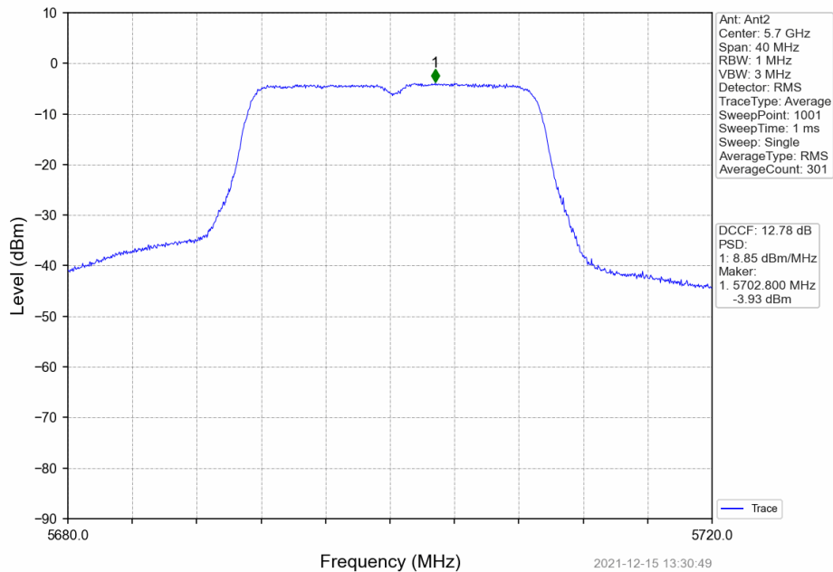
802.11n(HT20)_HCH_5700MHz_Ant2_NTNV
