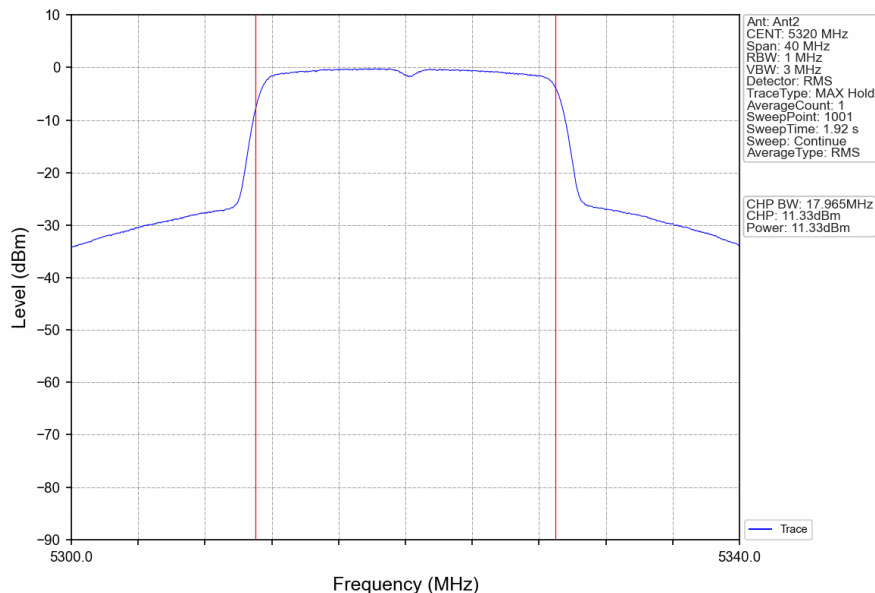
802.11n(HT20)_HCH_5320MHz_Ant2_NTNV
