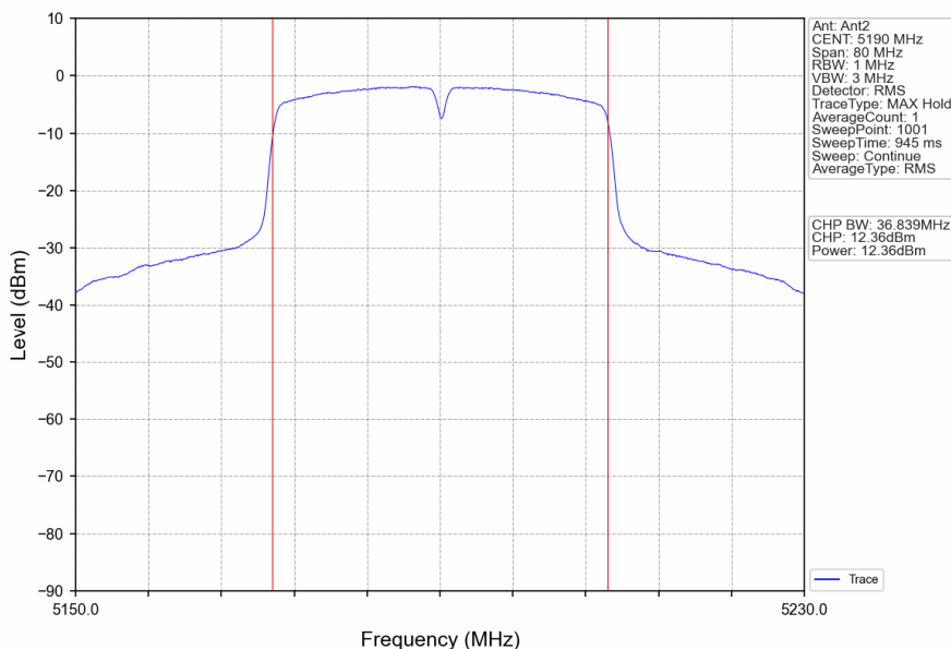
802.11n(HT40)_LCH_5190MHz_Ant2_NTNV
