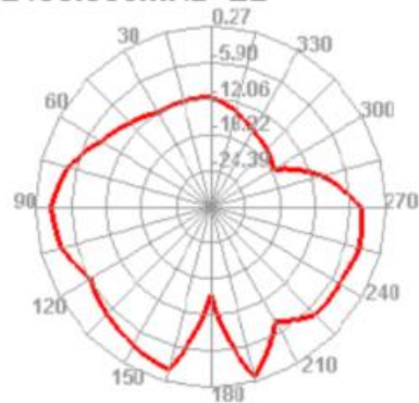
2400.000MHz E2
