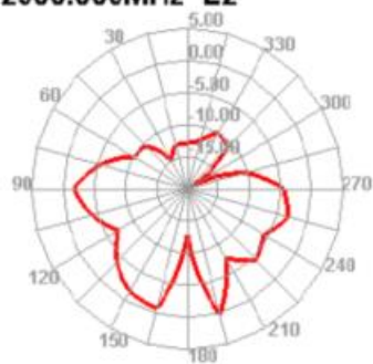
2500.000MHz E2
