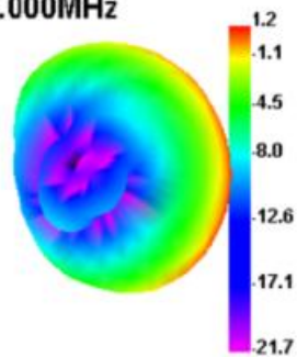
2500.000MHz
