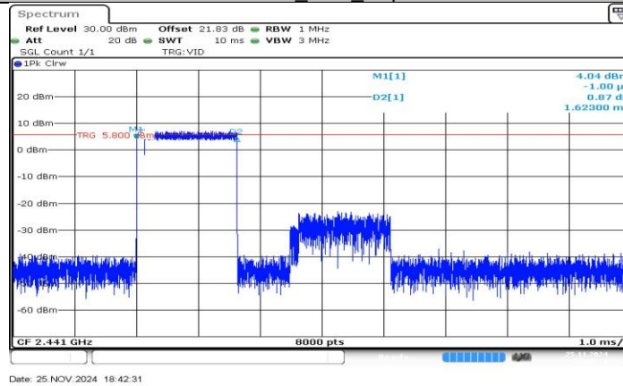
3DH3_Ant1_Hop
