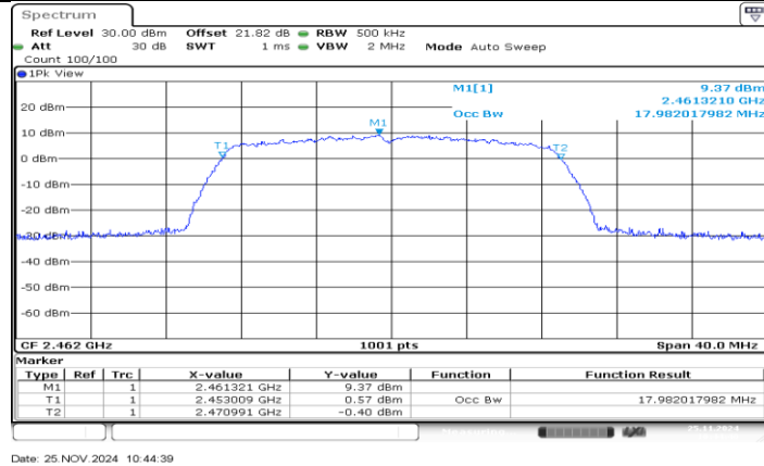
11N20MIMO_Ant2_2462
