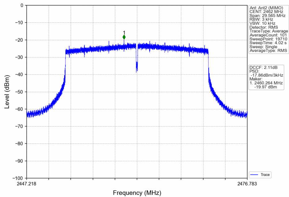
802.11ax(HEW20) HCH 2462MHz RU242 Left Ant2 (MIMO) NTV
