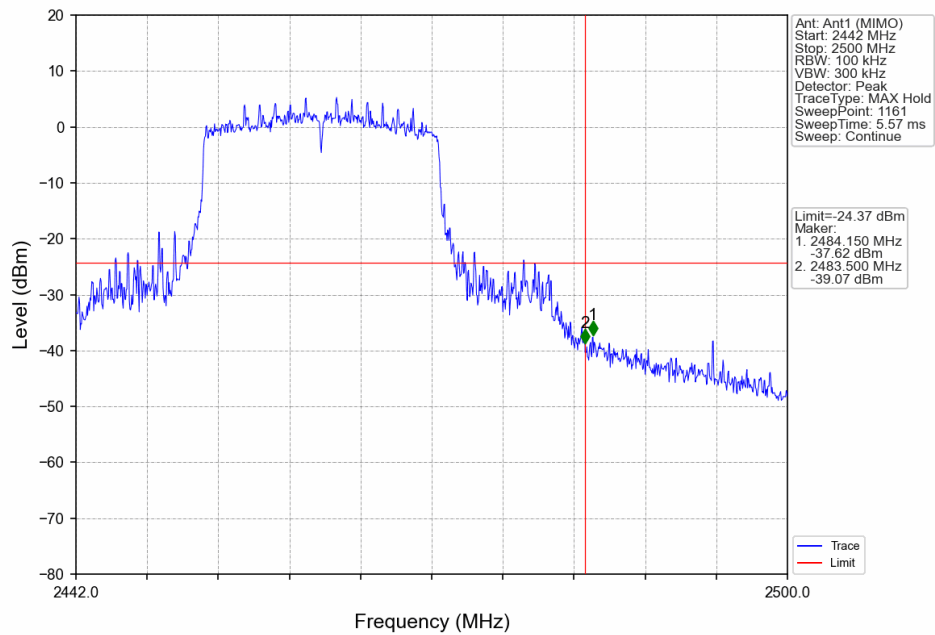
802.11ax(HEW20) HCH 2462MHz RU242 Left Ant1 (MIMO) NTVN
