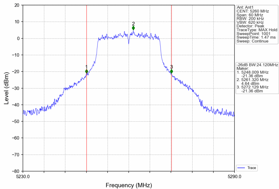
802.11n(HT20)_LCH_5260MHz_Ant1_NTN
