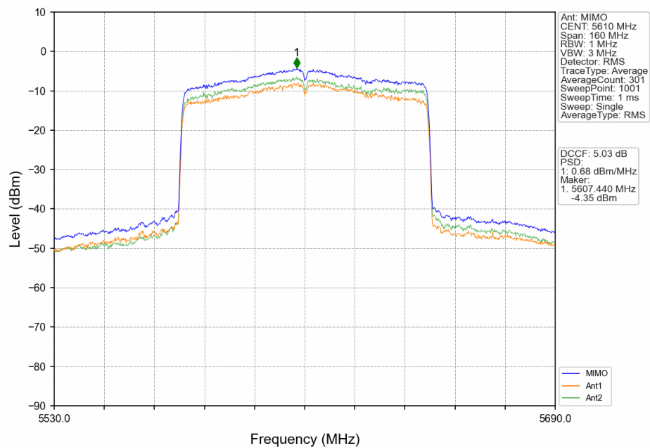
802.11ax(HEW80) HCH 5610MHz RU996 Left MIMO NTNv
