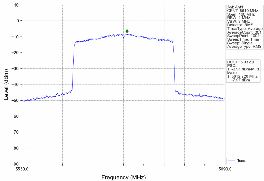
802.11ax(HEW80) HCH 5610MHz RU996 Left Ant1 NTNv
