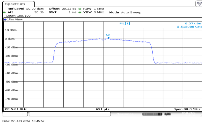
11AX40MIMO_Ant1_5510
