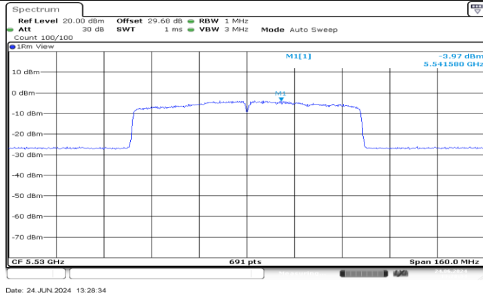
11AC80MIMO_Ant2_5530
