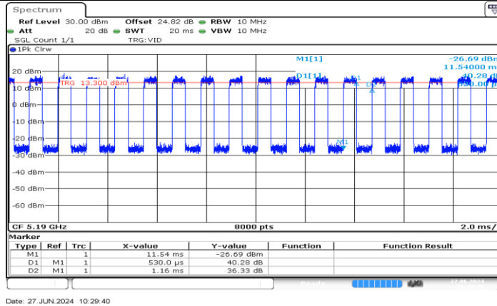
11AX40MIMO_Ant1_5190
