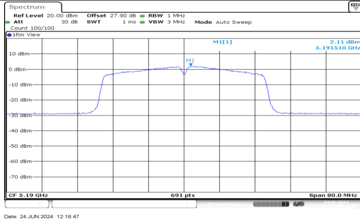
11N40MIMO Ant1 5190
