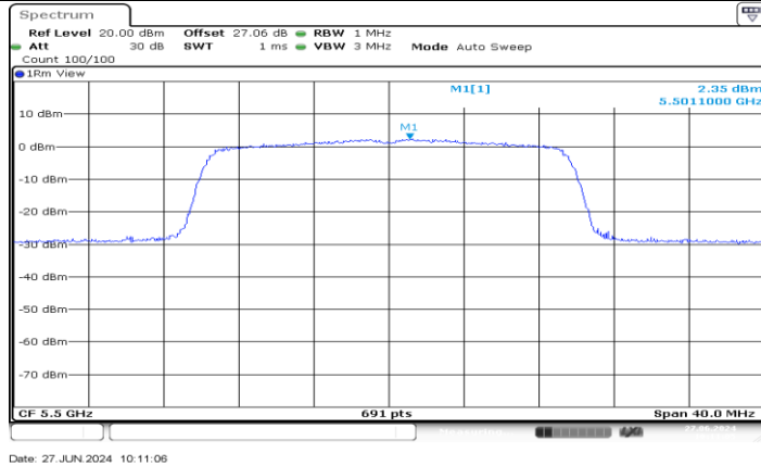
11AX20MIMO_Ant1_5500
