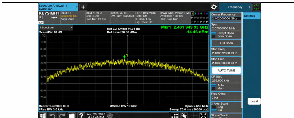
BLE 2M-Ant1-2402-PASS
