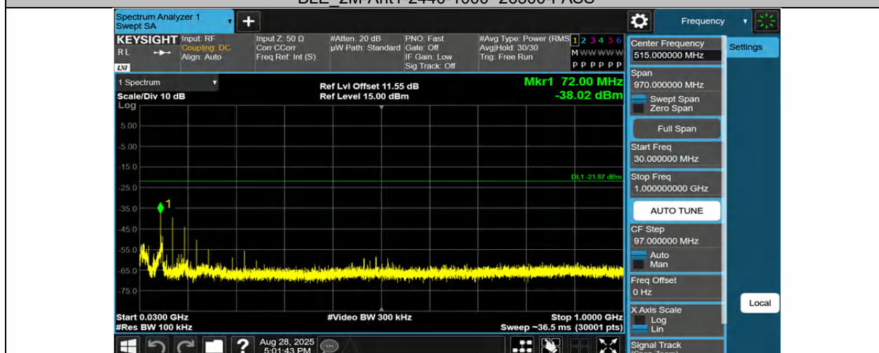
BLE_2M-Ant1-2480-30~1000-PASS
