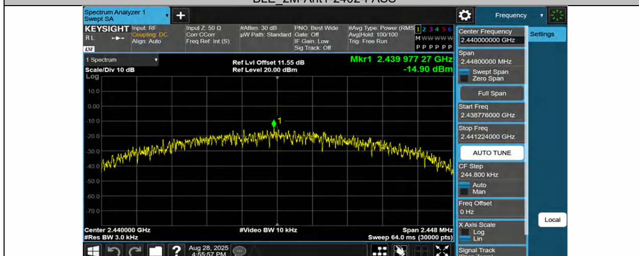
BLE 2M-Ant1-2440-PASS
