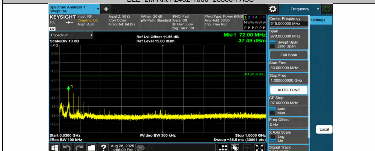
BLE_2M-Ant1-2440-30~1000-PASS
