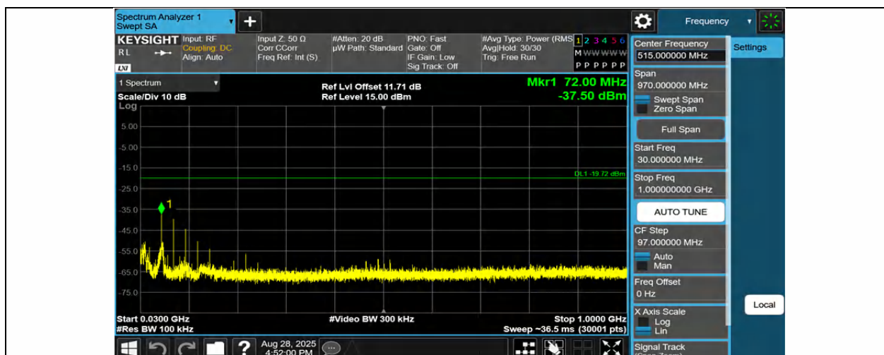
BLE_2M-Ant1-2402-30~1000-PASS
