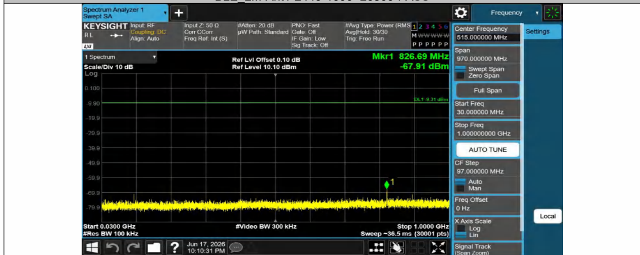
BLE_2M-Ant1-2480-30~1000-PASS
