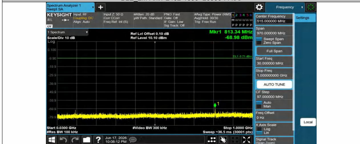
BLE_2M-Ant1-2440-30~1000-PASS
