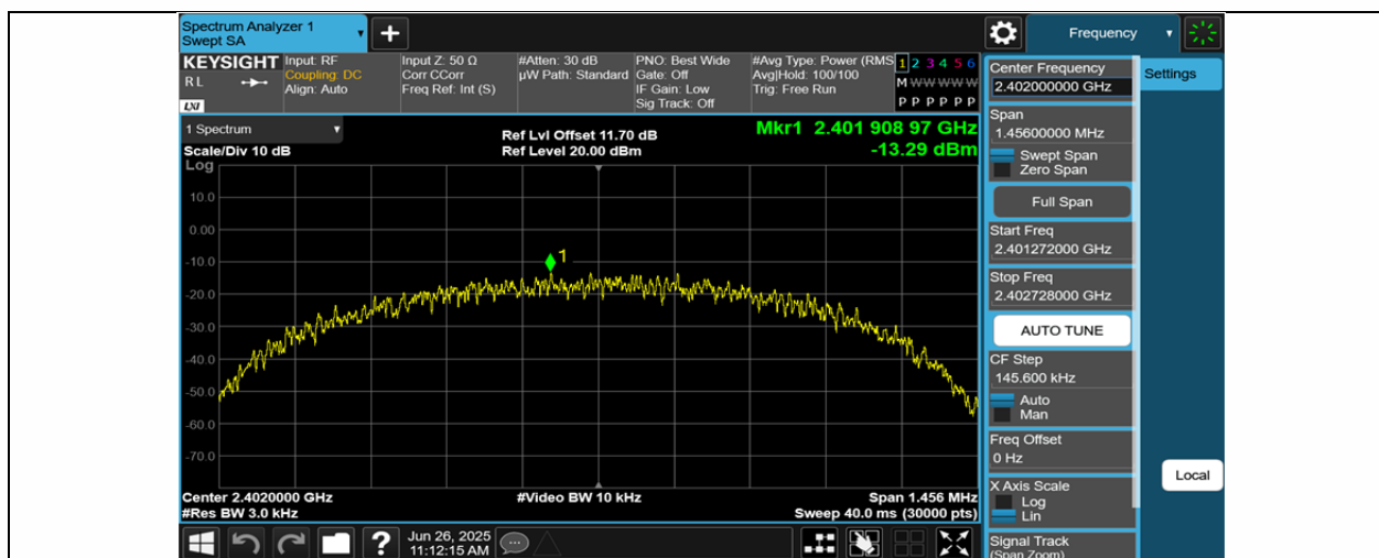
BLE 1M-Ant1-2402-PASS
