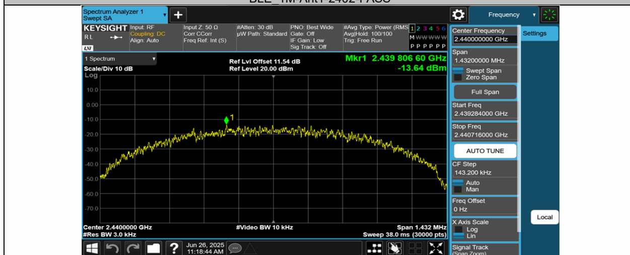
BLE 1M-Ant1-2440-PASS
