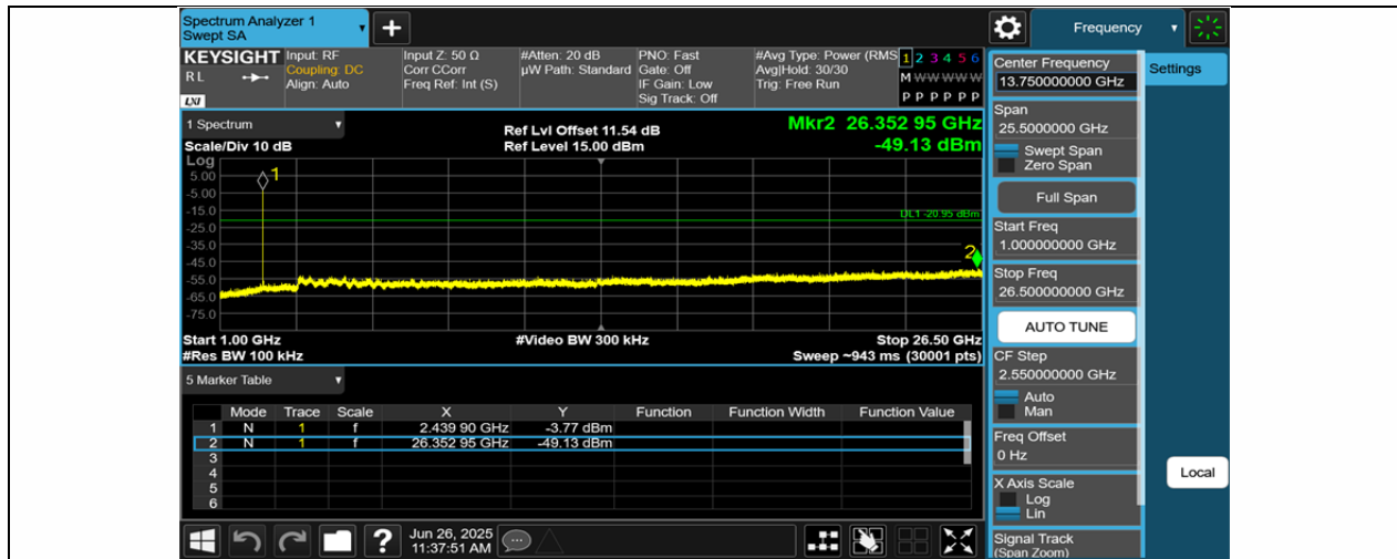
BLE 2M-Ant1-2440-1000~26500-PASS
