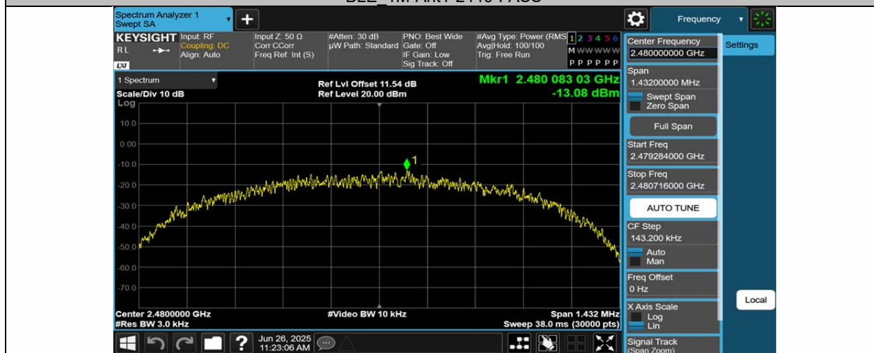
BLE 1M-Ant1-2480-PASS
