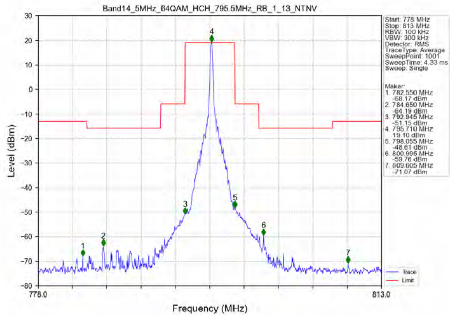
Band14 5MHz 64QAM HCH 795.5MHz RB 1 13 NTV
