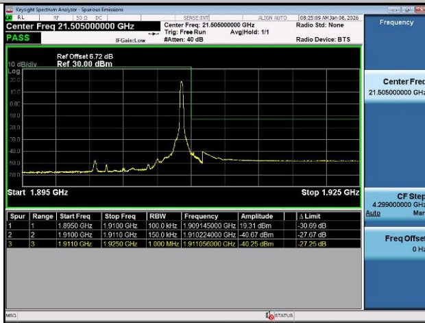
Band2-20MHz-QPSK-18700-1RB#0-PASS
