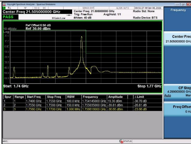
Band4-20MHz-QPSK-20050-1RB#0-PASS
