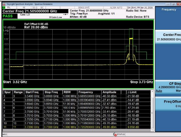
Band48-10MHz-QPSK-55290-1RB#49-PASS
