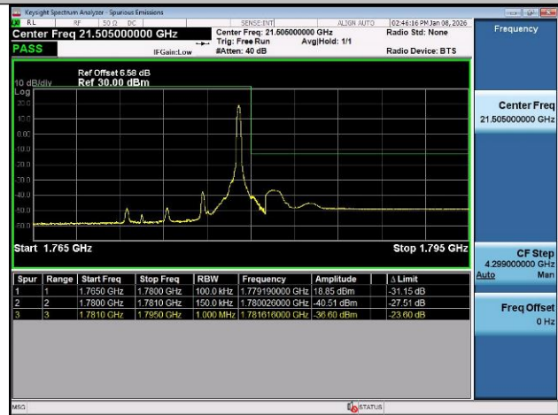
Band66-20MHz-QPSK-132072-1RB#0-PASS
