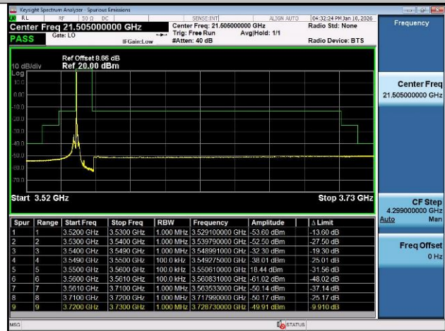
Band48-10MHz-QPSK-55290-50RB#0-PASS
