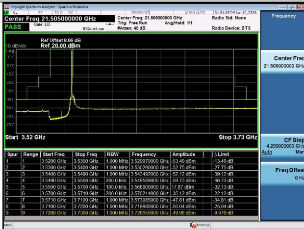
Band48-20MHz-QPSK-56640-1RB#0-PASS
