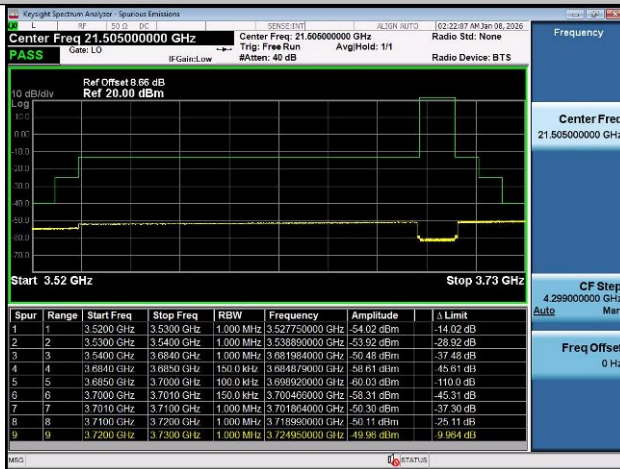
Band48-20MHz-QPSK-55340-1RB#99-PASS
