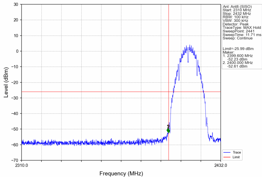
802.11b_LCH_2412MHz_Ant8 (SISO)_NTNV
