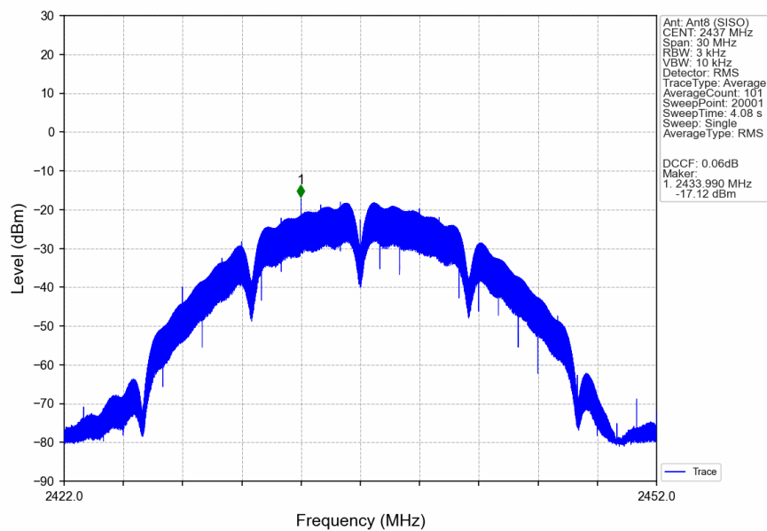
802.11b_MCH_2437MHz_Ant8 (SISO)_NTNV
