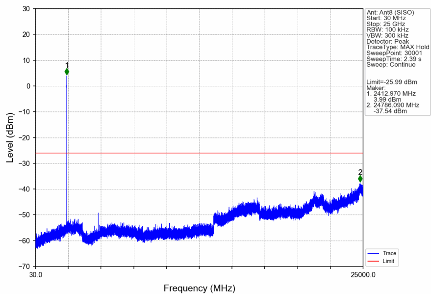
802.11b_LCH_2412MHz_Ant8 (SISO)_NTNV
