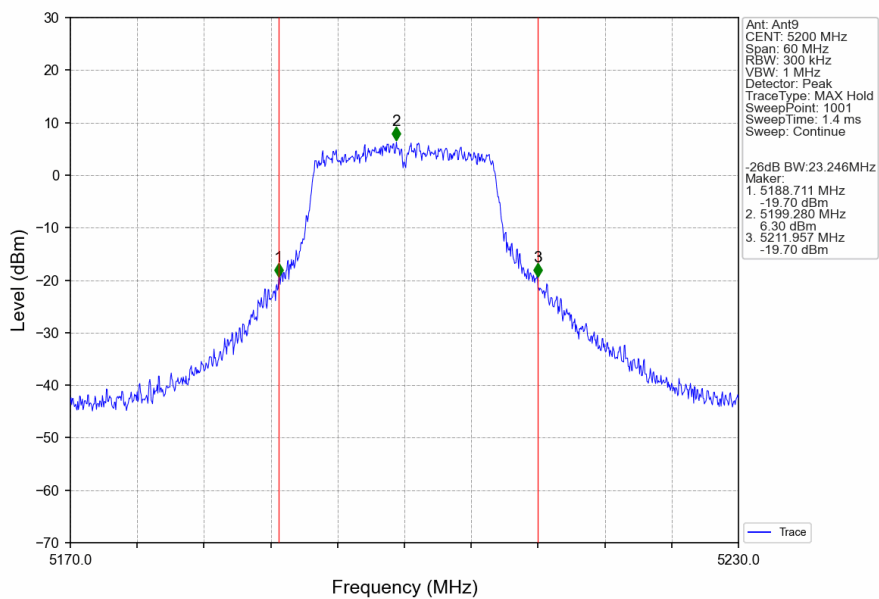
802.11a_MCH_5200MHz_Ant9_NTNV
