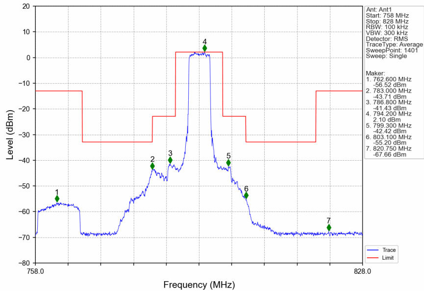
Band14_10MHz_QPSK_MCH_793MHz_RB_25_25_NTNV
