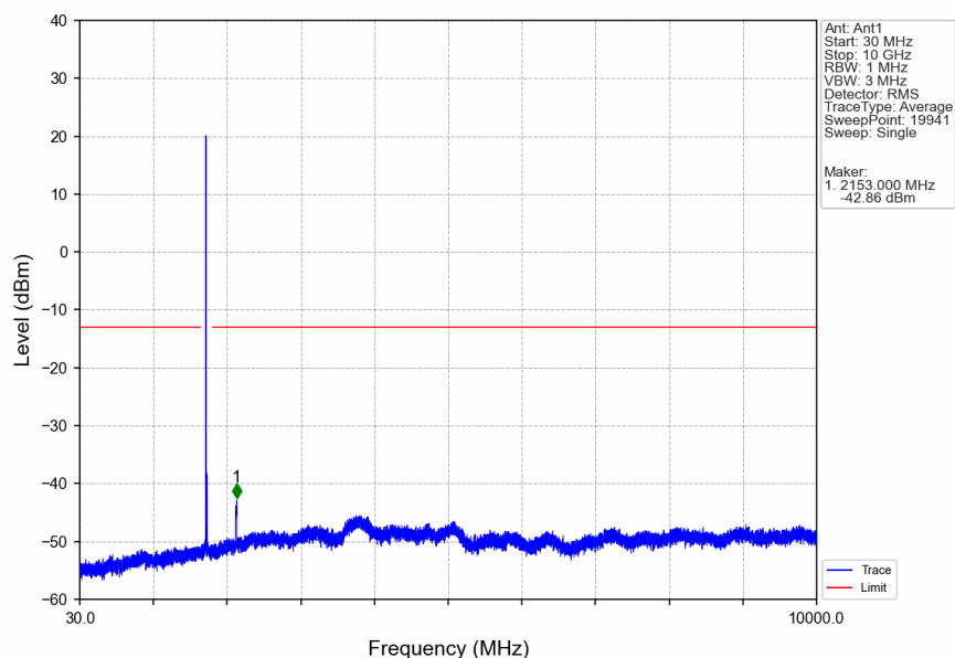
Band66_20MHz_QPSK_MCH_1745MHz_RB_1_0_NTNV
