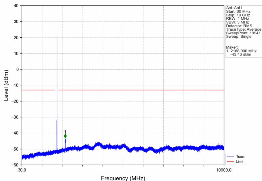
Band66_20MHz_QPSK_HCH_1770MHz_RB_1_0_NTNV
