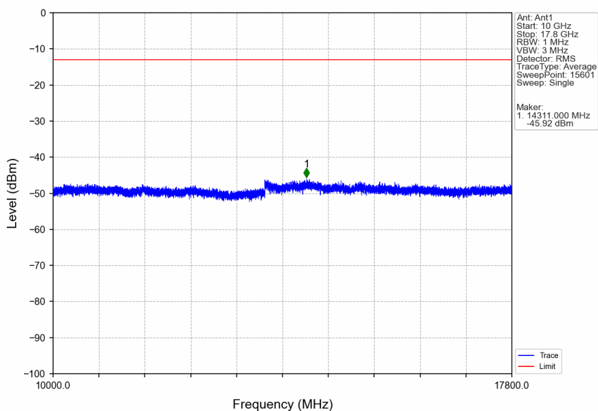
Band66_20MHz_QPSK_HCH_1770MHz_RB_1_0_NTNV
