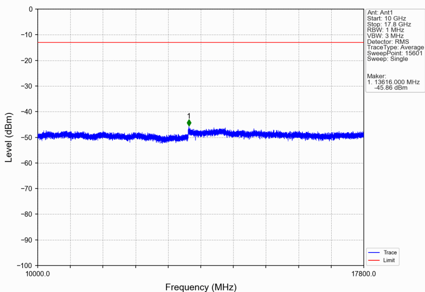
Band66_20MHz_QPSK_MCH_1745MHz_RB_1_0_NTNV
