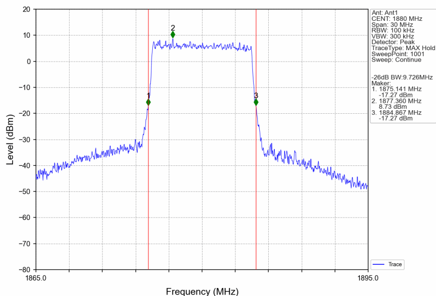
Band2_10MHz_256QAM_MCH_1880MHz_RB_50_0_NTNV
