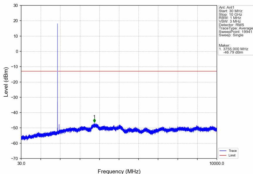
Band2_1.4MHz_QPSK_MCH_1880MHz_RB_1_0_NTNV
