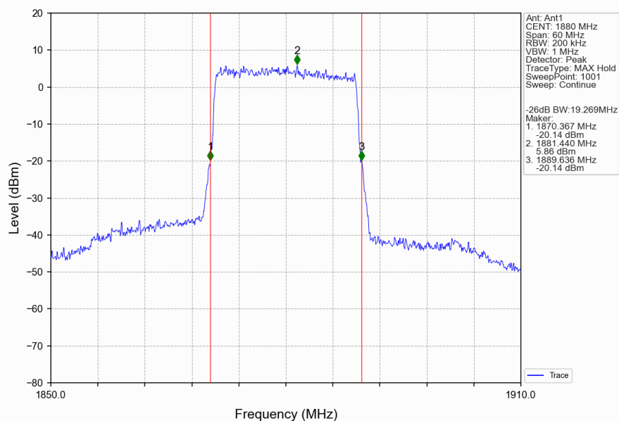
Band2_20MHz_256QAM_MCH_1880MHz_RB_100_0_NTNV
