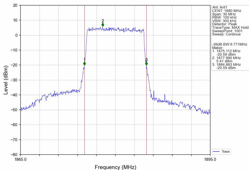
Band2_10MHz_256QAM_MCH_1880MHz_RB_50_0_NTNV
