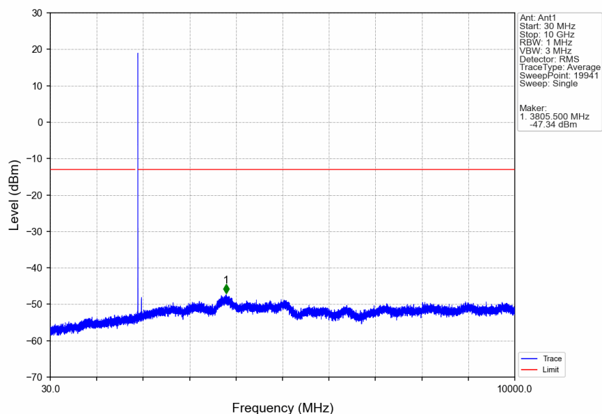
Band2_1.4MHz_QPSK_HCH_1909.3MHz_RB_1_0_NTNV
