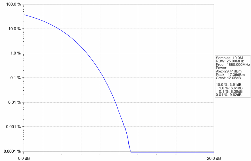
Band2_20MHz_64QAM_MCH_1880MHz_RB_100_0_NTNV
