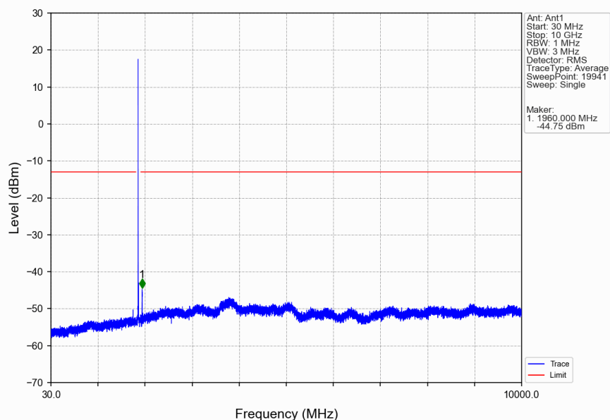
Band2_10MHz_QPSK_MCH_1880MHz_RB_1_0_NTNV
