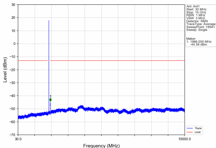
Band2_20MHz_QPSK_MCH_1880MHz_RB_1_0_NTNV
