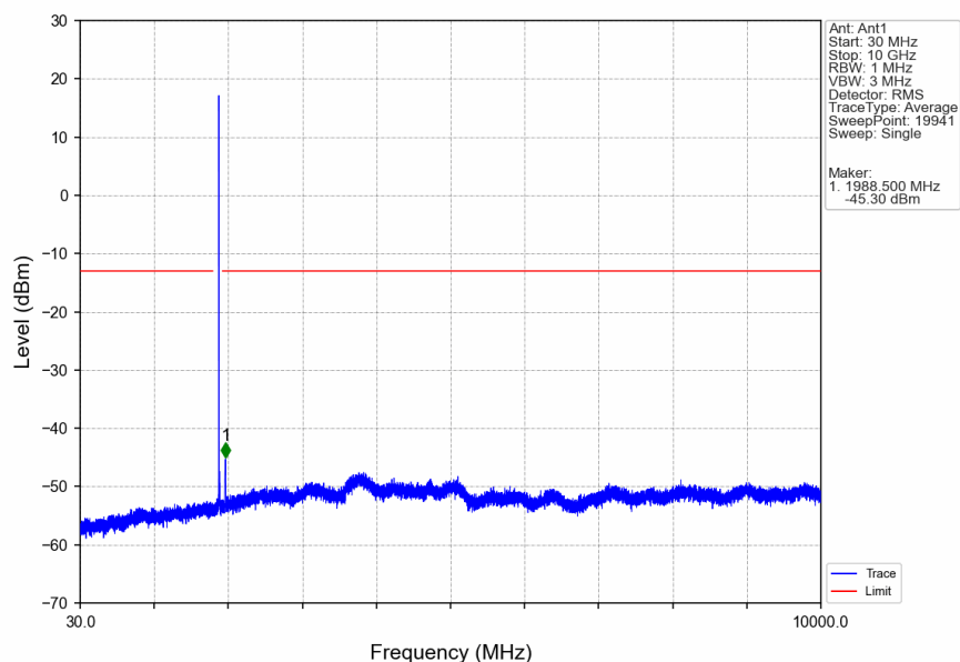
Band2_15MHz_QPSK_HCH_1902.5MHz_RB_1_0_NTNV
