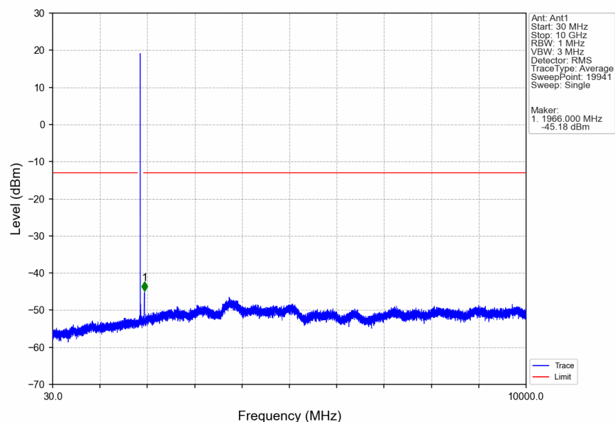
Band2_15MHz_QPSK_MCH_1880MHz_RB_1_0_NTNV
