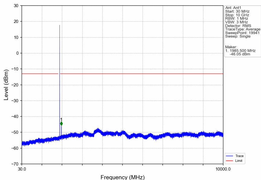
Band2_10MHz_QPSK_HCH_1905MHz_RB_1_0_NTNV
