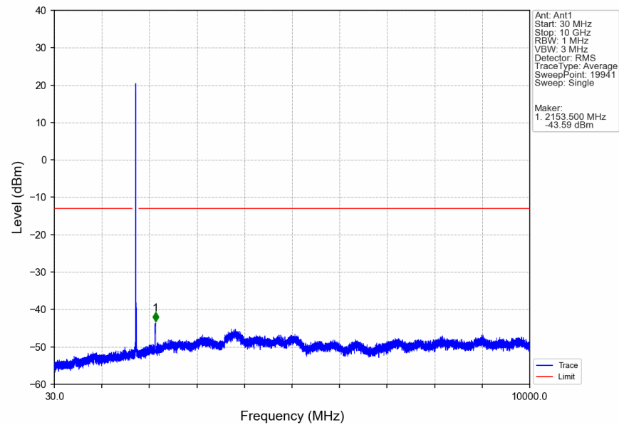
Band4_20MHz_QPSK_HCH_1745MHz_RB_1_0_NTNV
