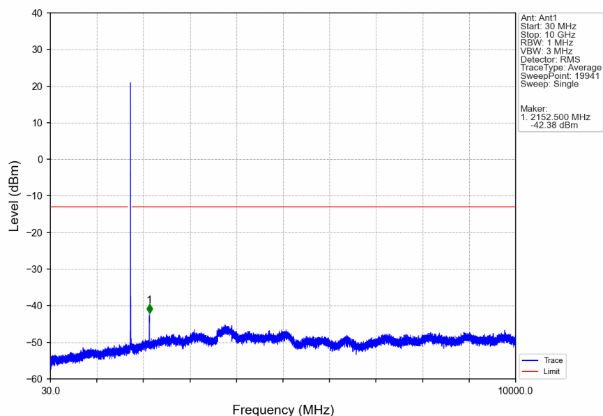
Band4_10MHz_QPSK_HCH_1750MHz_RB_1_0_NTNV
