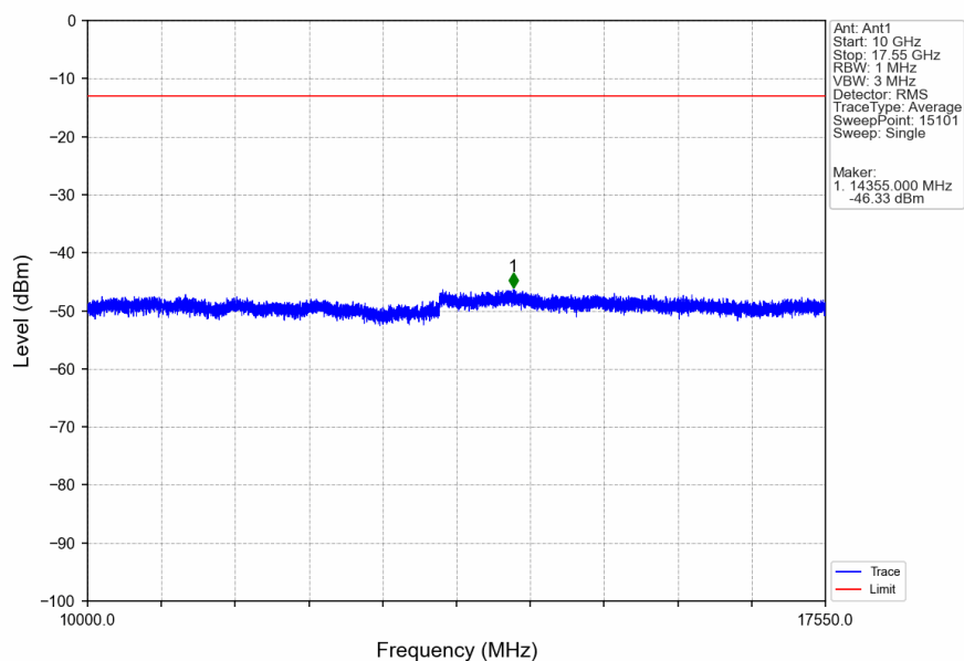
Band4_10MHz_QPSK_HCH_1750MHz_RB_1_0_NTNV
