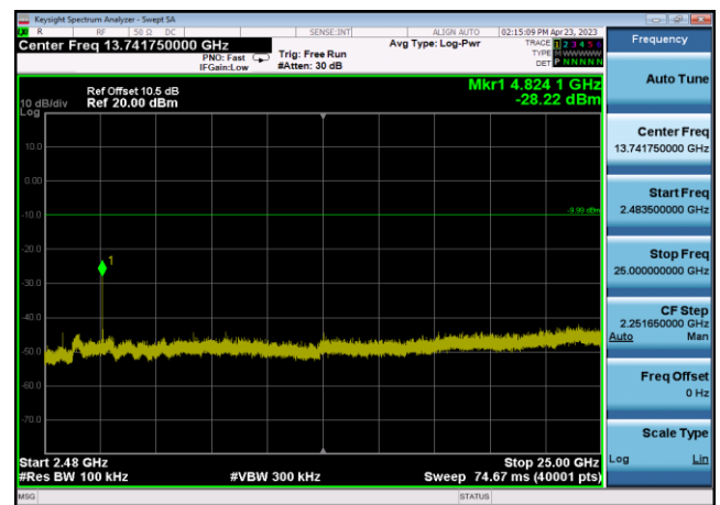
,Plot 4,2483.5MHz~25000MHz-802.11b
