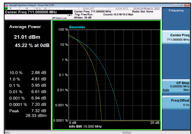
FDD12_HighRange_10MHz_711_fullIRB _Q16
