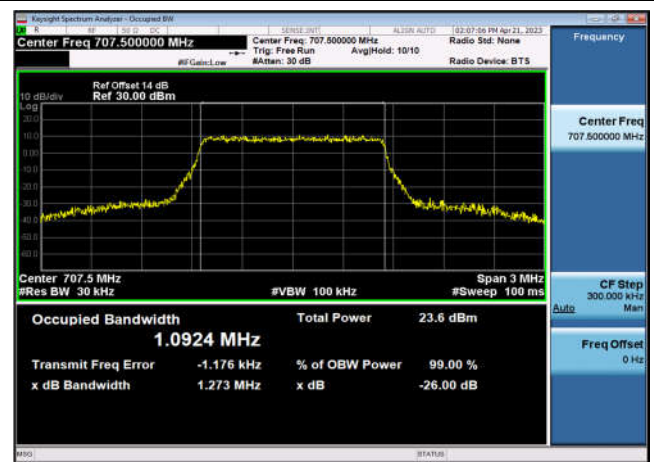
FDD12_MidRange_3_707.5_Q16
