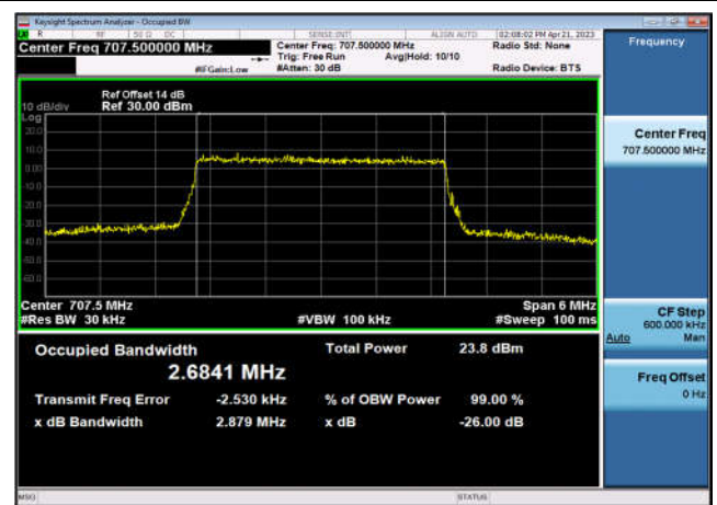
FDD12_MidRange_3_707.5_Q16
