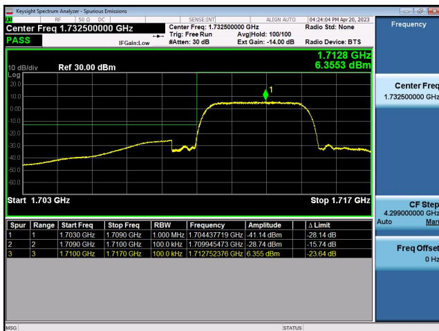
WCDMA 1700-1312
