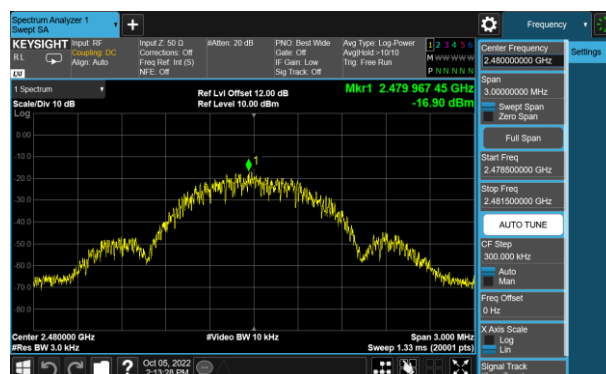
LE CH39 (2480MHz)
