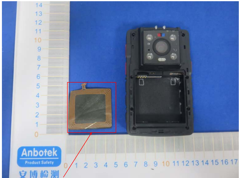
NFC ANT
