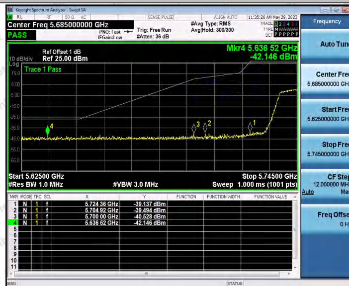
11N40ISO_Ant2_Low_5755
