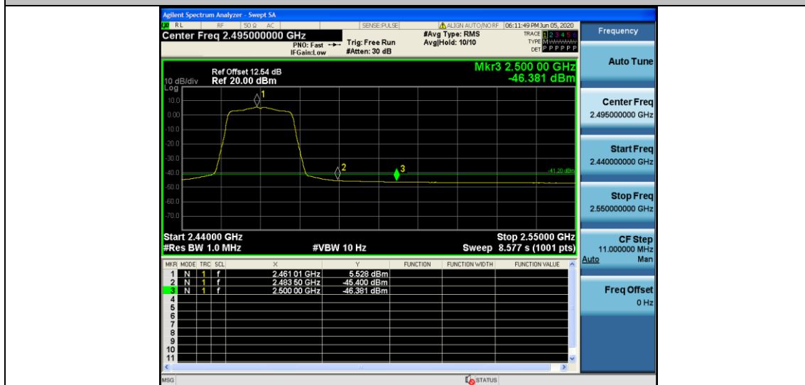
11N20MIMO_Ant1_High_2462_AV
