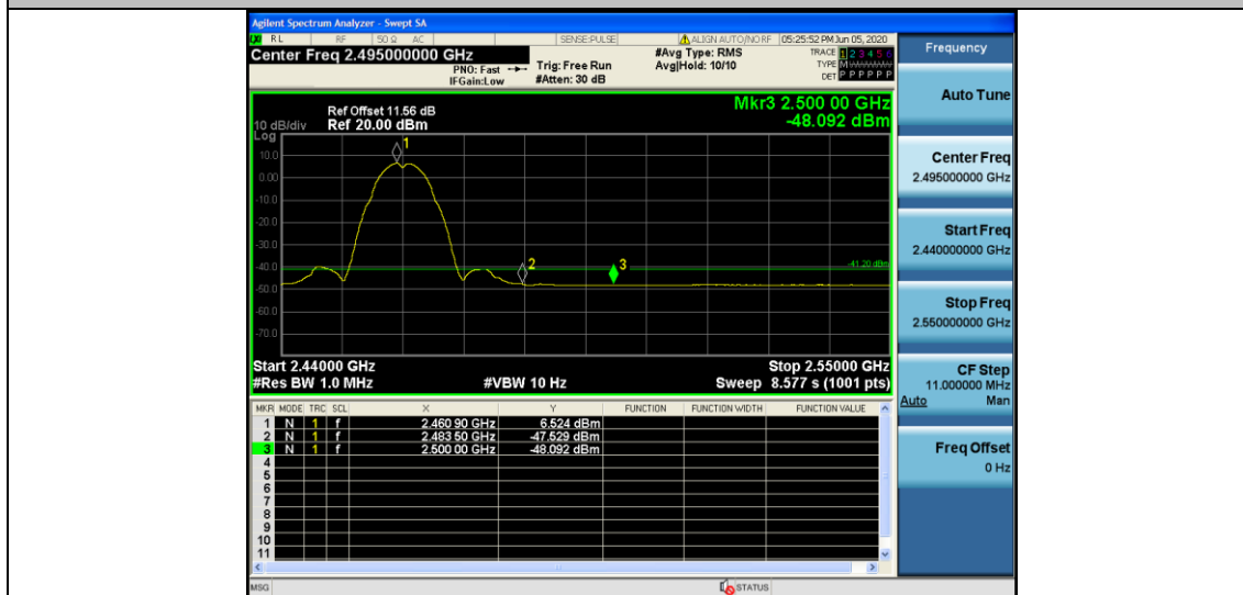
11B_Ant0_High_2462_AV
