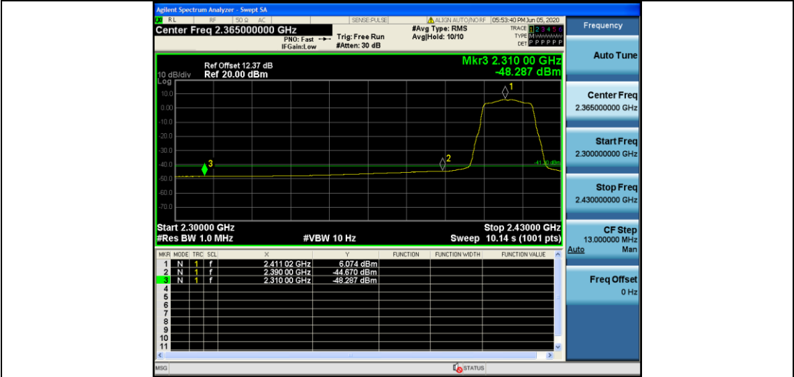
11G_Ant1_Low_2412_AV
