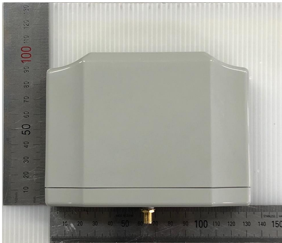
RFID Antenna 4 (M/N: MACRO130-919)
