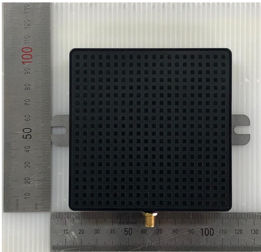
RFID Antenna 5 (M/N: MACRO100-919)
