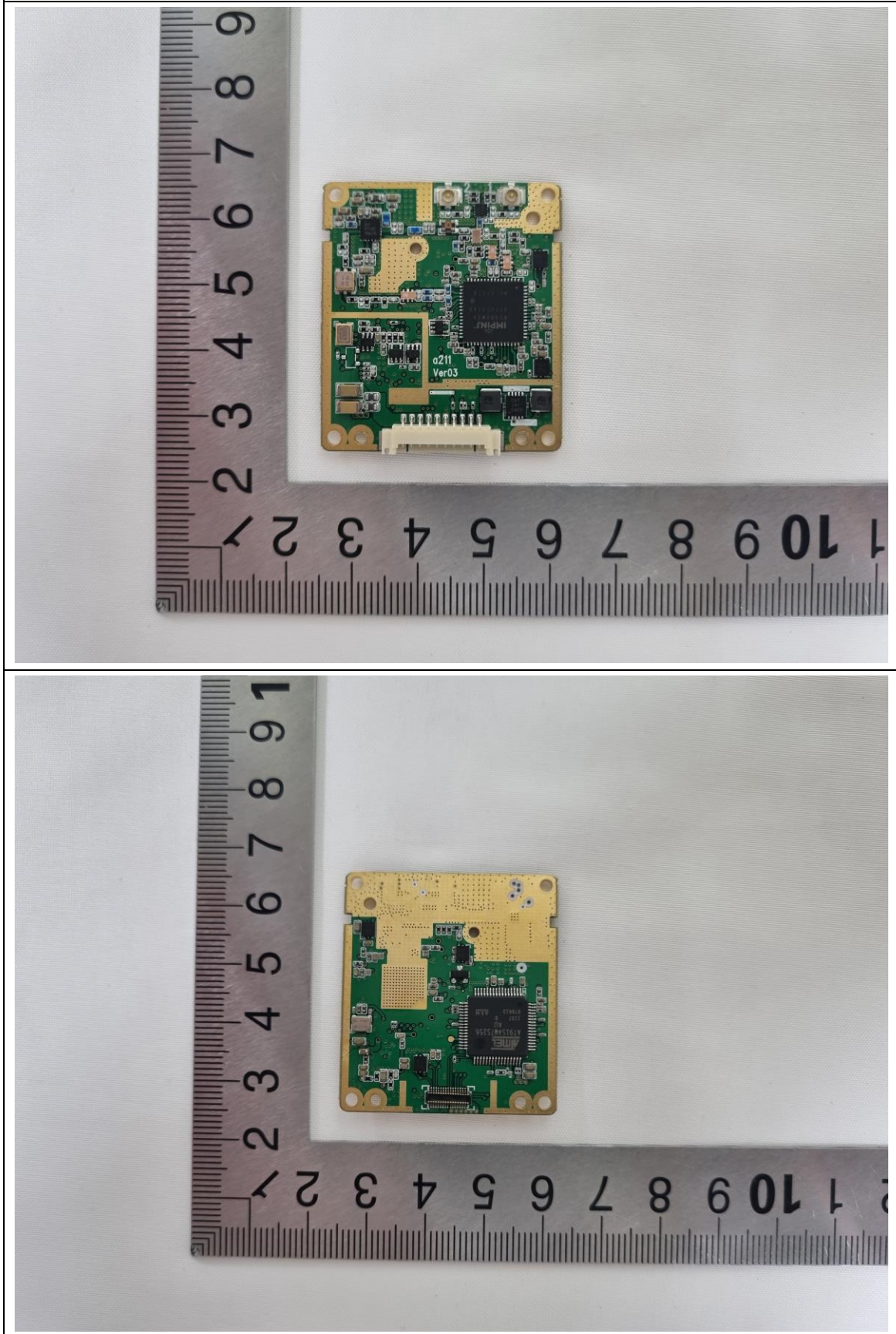
RFID Module
