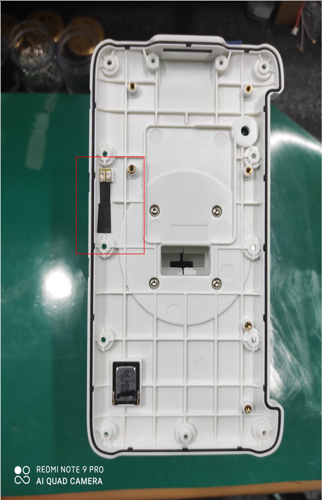
ANTENNA(2.4 GHz)
