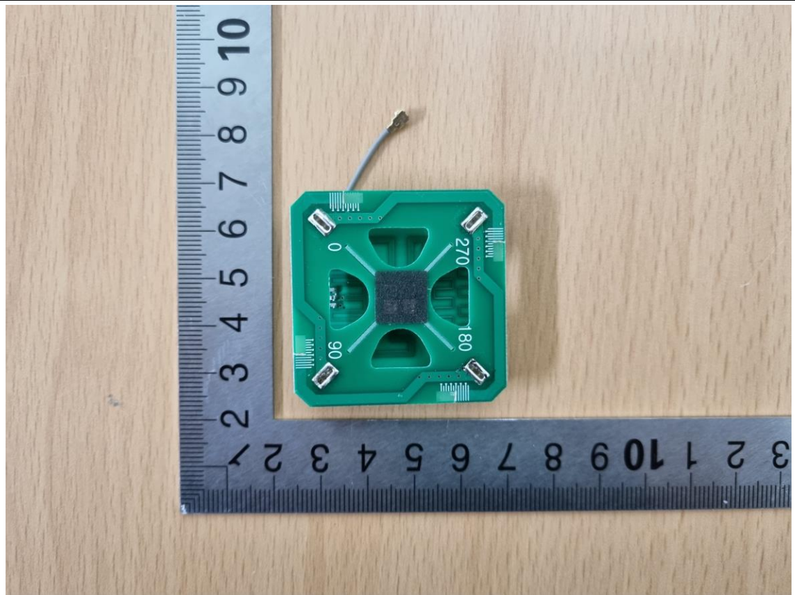
RFID Antenna
