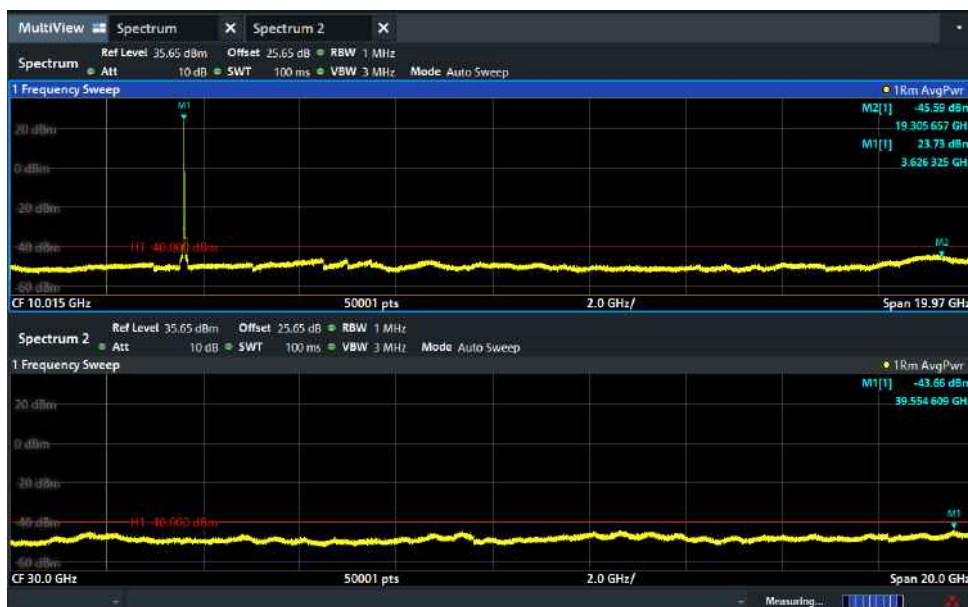
10 MHz_641666_1.1_CSE_Ant2
