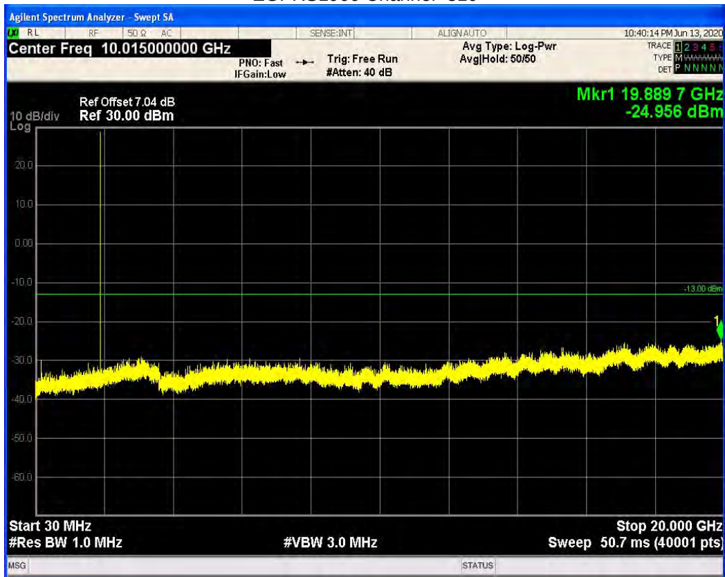
EGPRS1900 Channel=810
