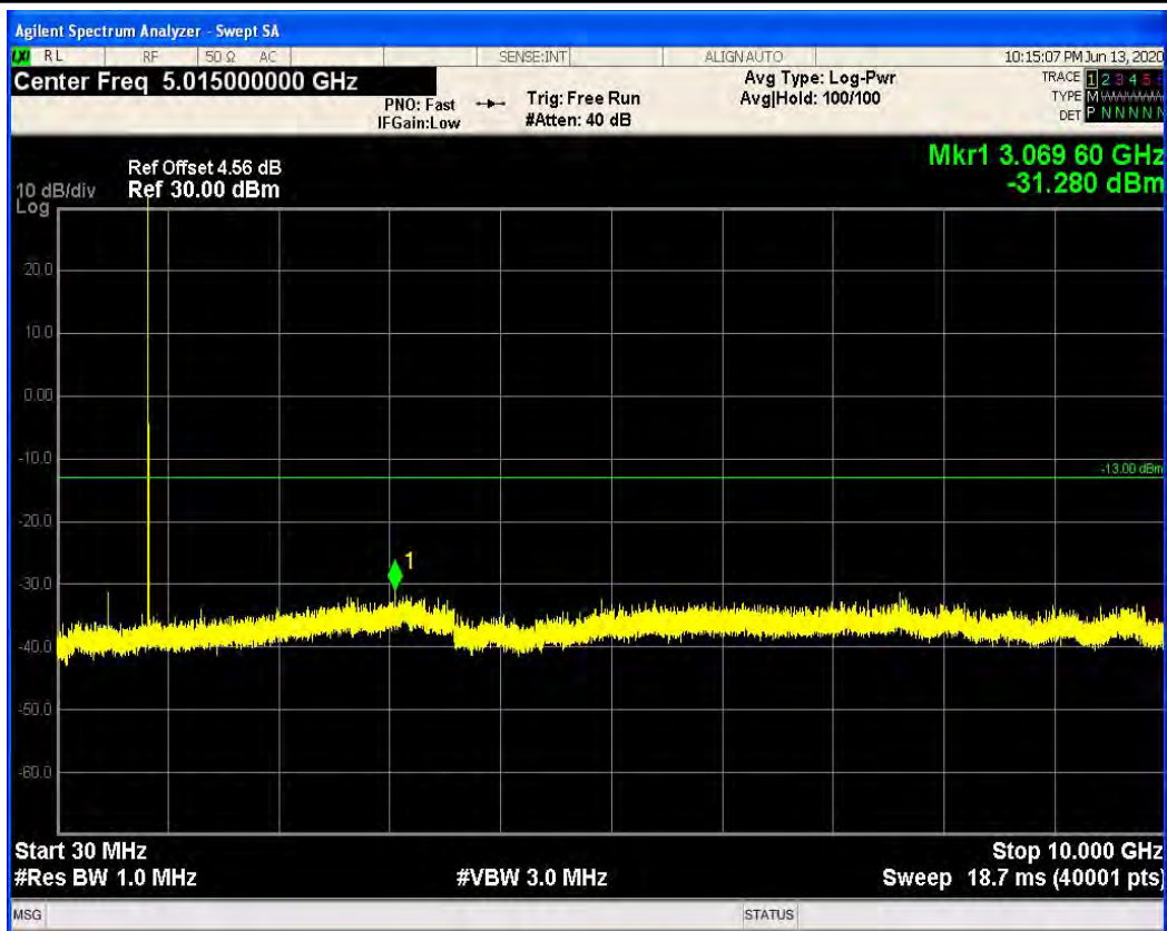
EGPRS1900 Channel=512
