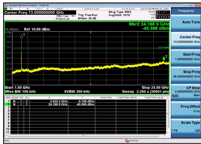
1GHz-25GHz
