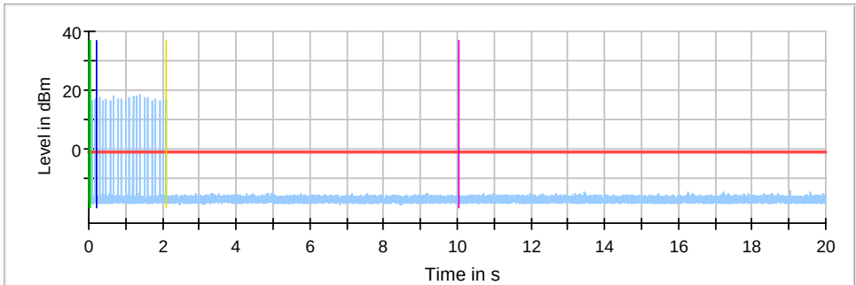
802.11ac VHT80 5610MHz
