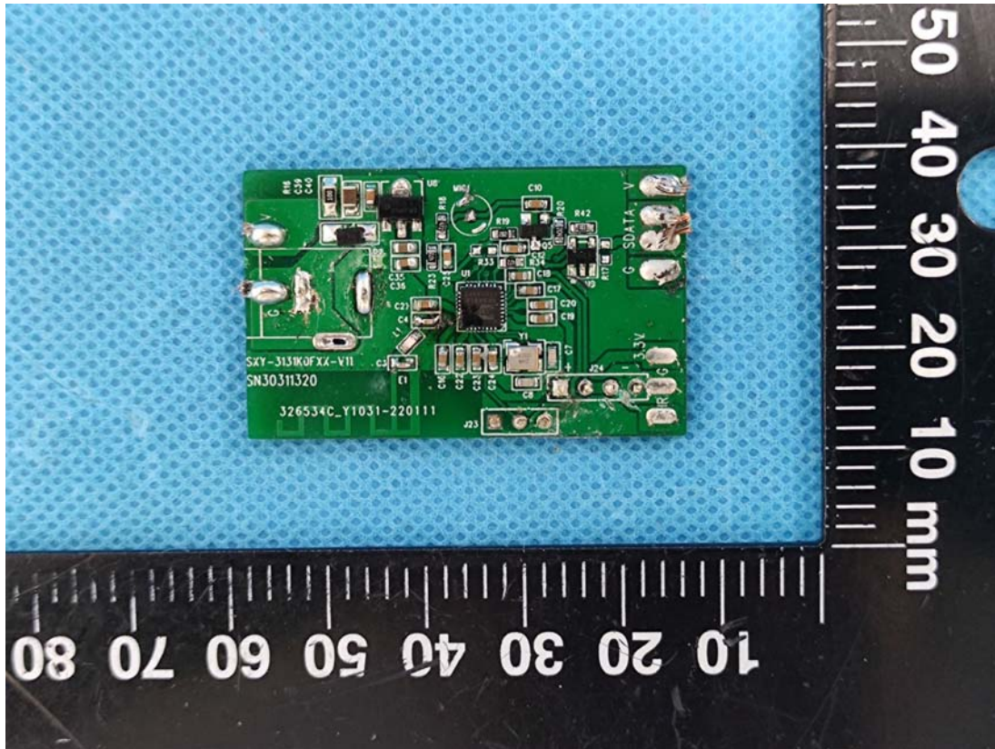
BLE Board
