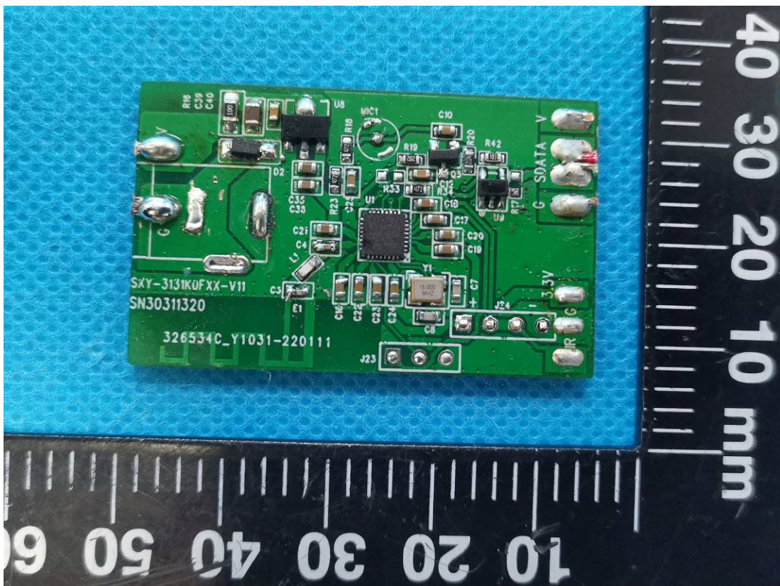
BLE Board
